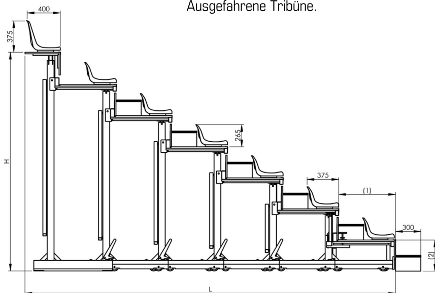
Ausgefahrene Tribüne.
