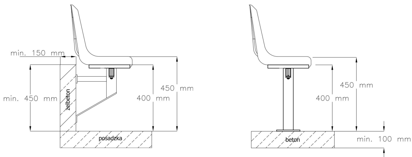
Hängende Befestigung
