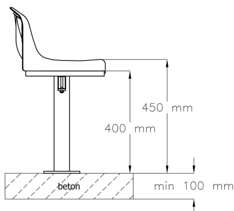
Stehende Befestigung
